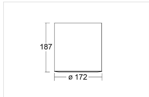
Afmetingen versie 2022
